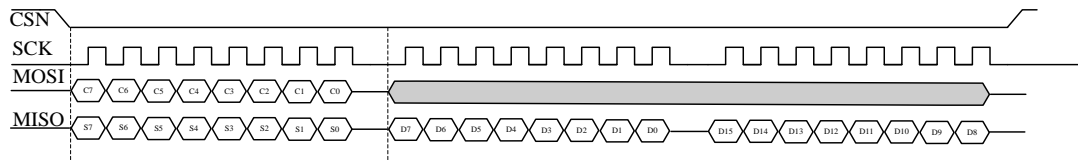
图5. SPI读操作
