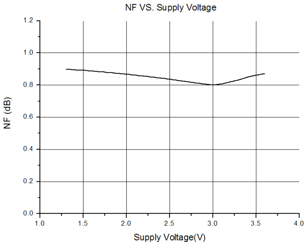
图一、噪声系数与供电电压的曲线
