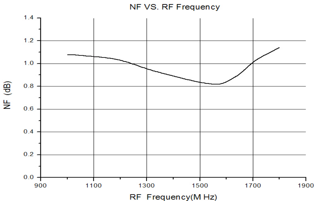
图二、噪声系数与工作频率的曲线
