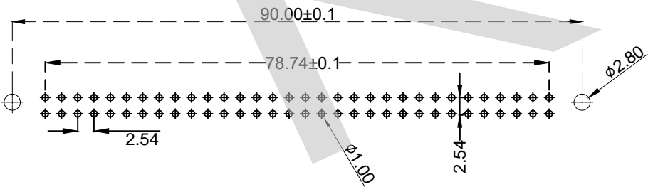
P.C.B LAYOUT
