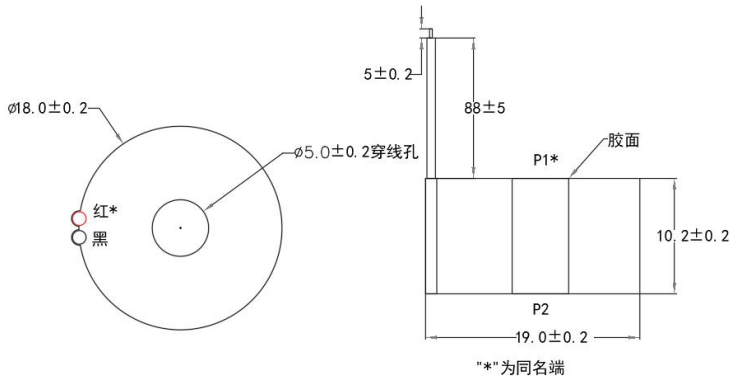
主视图
