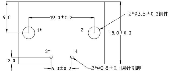
底视图
