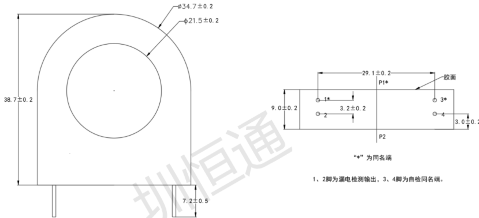
主视图
