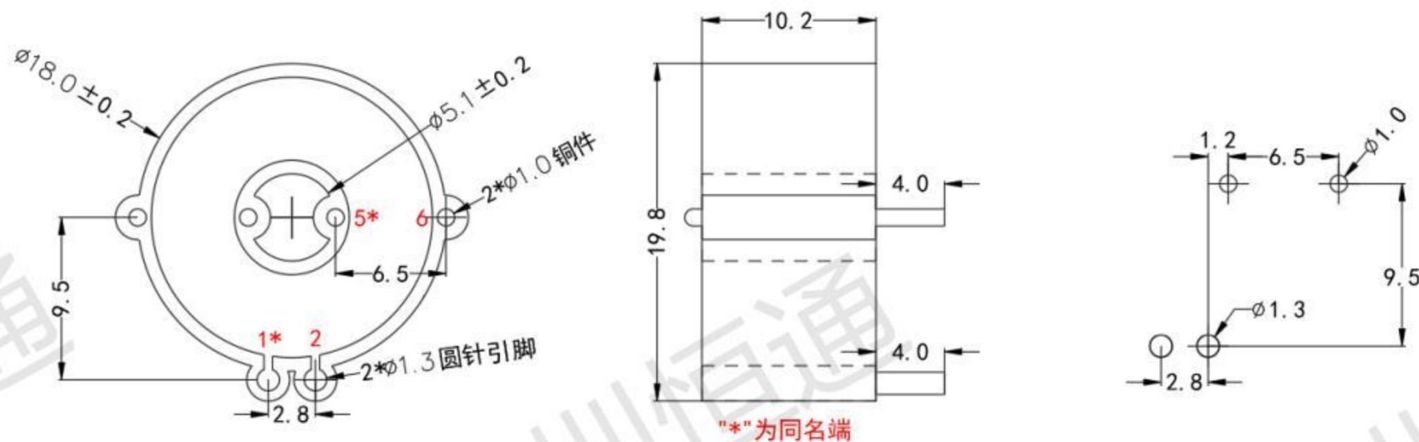
主视图
