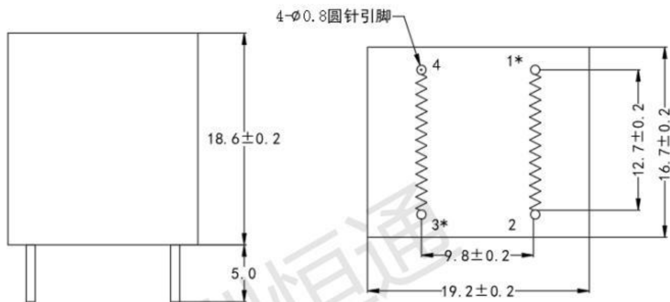
"*"为同名端 备注：尺寸允许误差范围±0.2
