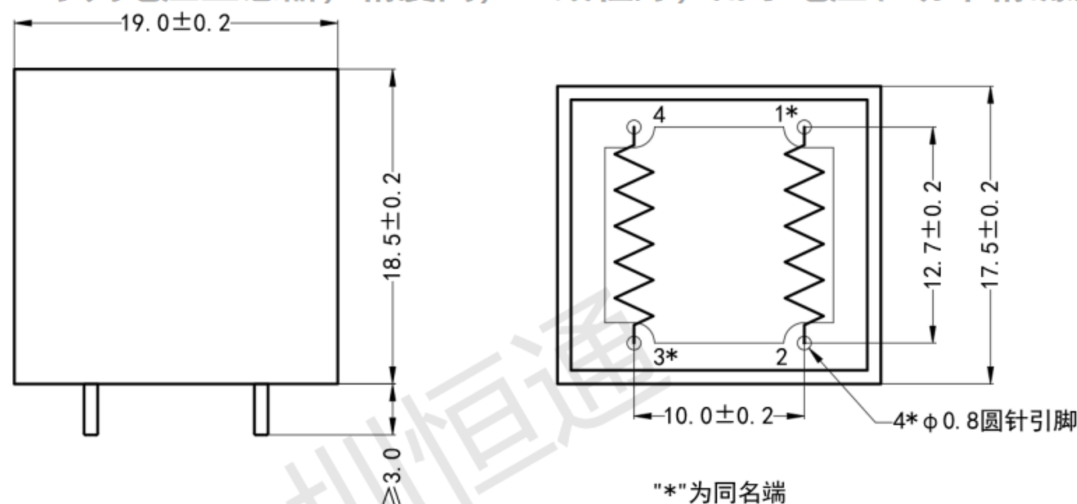
主视图
